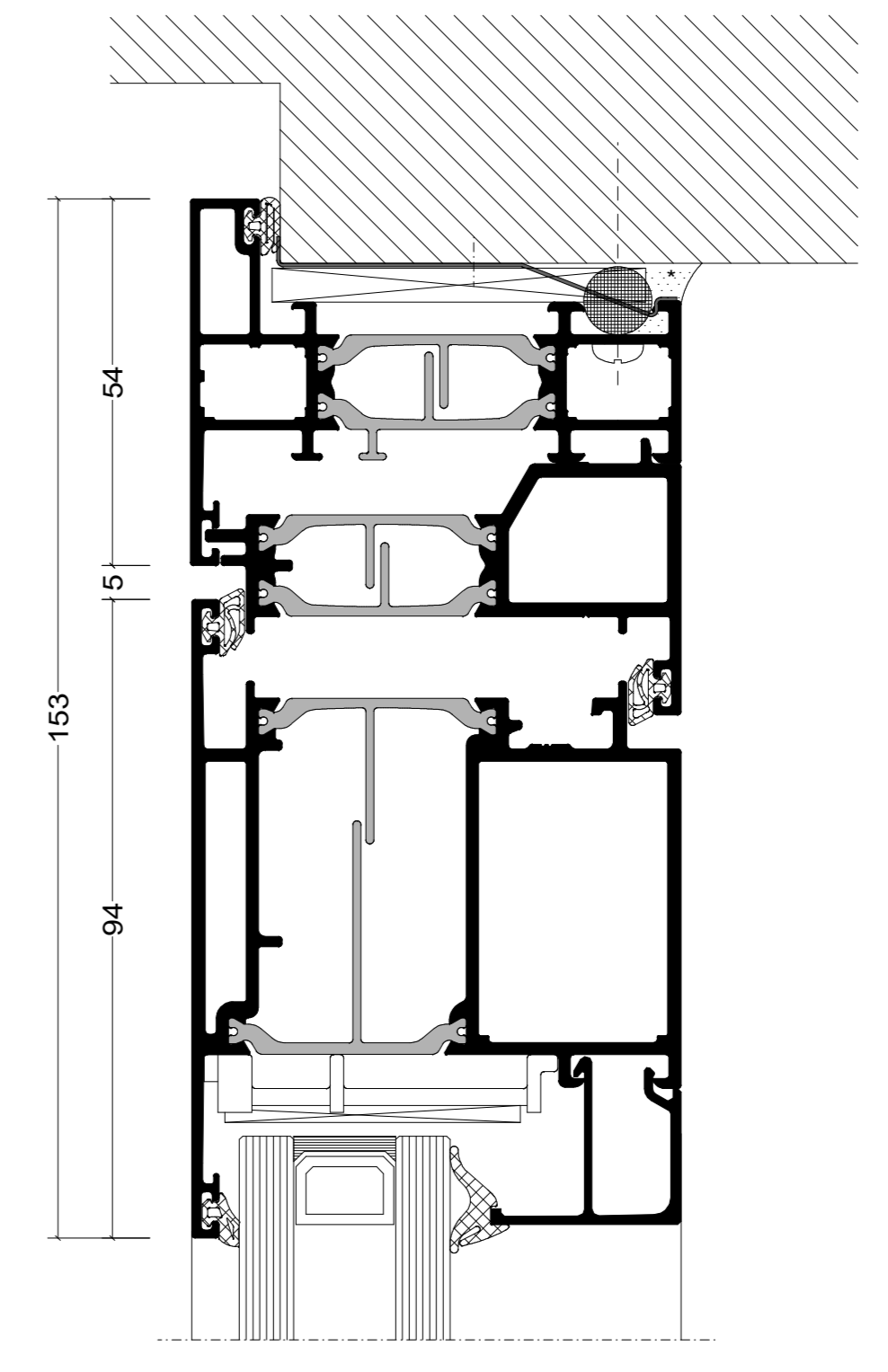
AANSLUITING BOVEN
