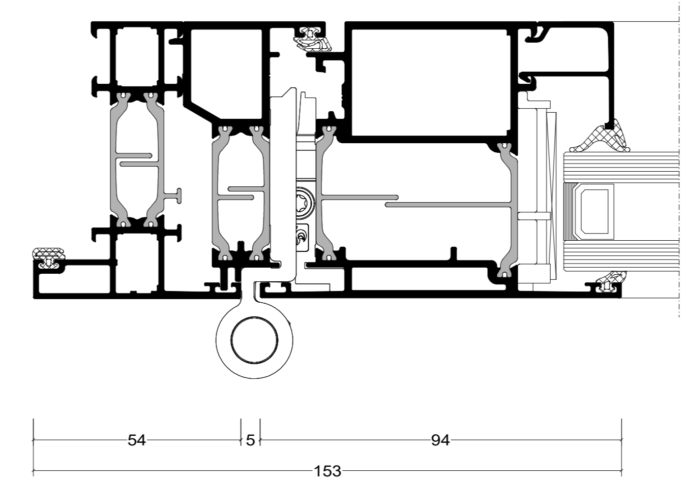
DUBBEL GLAS
